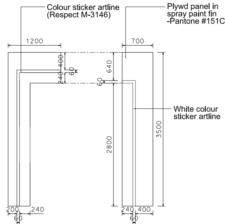
FASCIA ELEVATION
